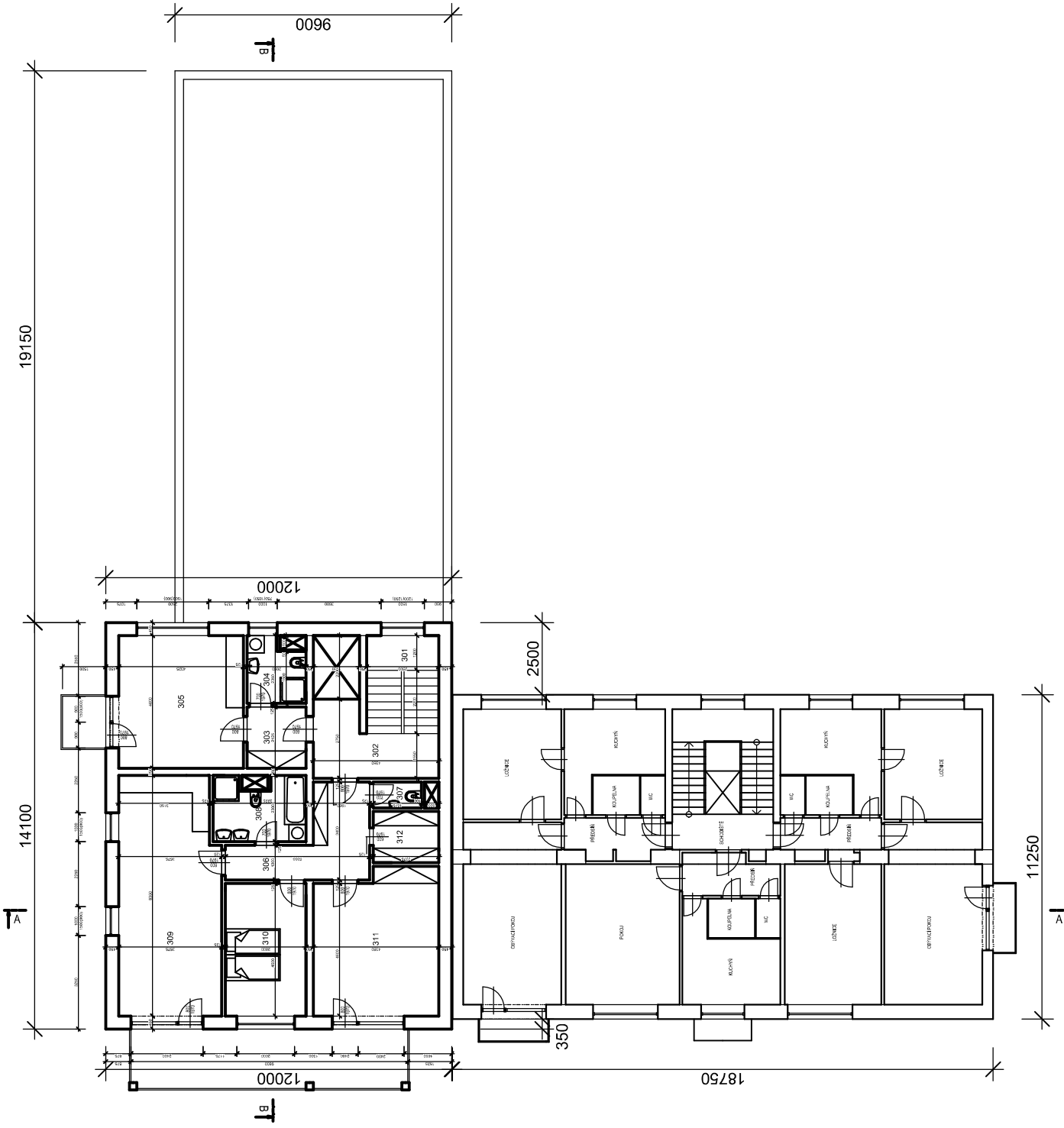
STÁVAJÍCÍ BD U CIHELNY 7 - 3.-7.NP - TYPICKÉ PODLAŽÍ
