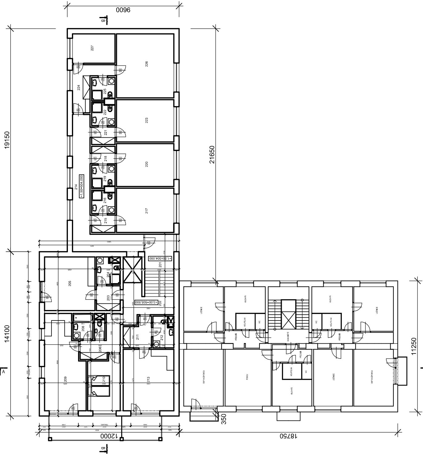
STÁVAJÍCÍ BD U CIHELNY 7 - 2.NP - TYPICKÉ PODLAŽÍ
